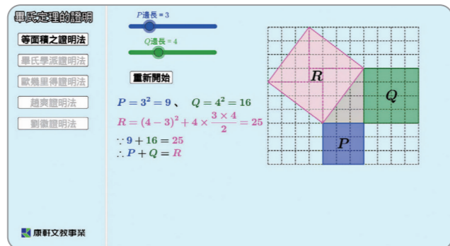
國中數學畢氏定理的證明程式
